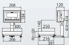
特設会社クボタ計装 特設会社クボタ (国産計装標準ユニット) 画像は、MS型計量台の外観参考図です。
