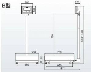
株式会社クボタ計装 株式会社クボタ (国産計装事業本部) 画像は、B型計量台の外観参考図です。
