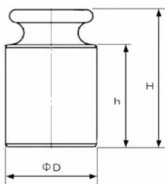
分銅外径図
