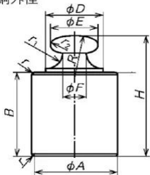
分銅外径図
