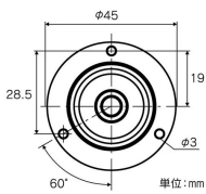
シムワ 測定株式会社 画像は、商品の外観参考寸法図です。
