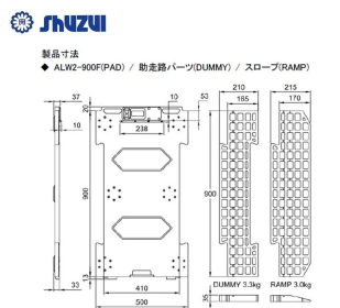
画像は、PADの寸法図です。
