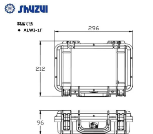
画像は、指示計：データBOXの寸法図です。
