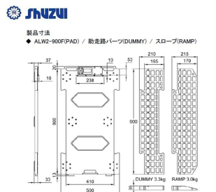
画像は、PADの寸法図です。
