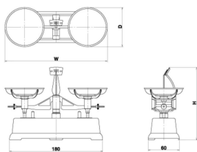
寸法図
