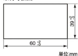
取付寸法図
