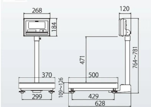
特約会社クボタ計装 特約会社クボタ (国産計装標準ユニット) 画像は、A型計量台の外観参考図です。
