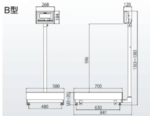
特約会社クボタ計装 画像は、B型計量台の外観参考図です。
