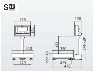
特約会社クボタ計装 特約会社クボタ (国産計装計器事業ユニット) 画像は、S型計量台の外観参考図です。
