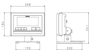
株式会社クボタ計装 株式会社クボタ (商品規格書第2.0.0版) 画像は、据置台の外観参考図です。
