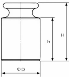
分銅外径図
