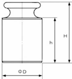
分銅外形図
