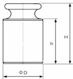
分銅外径図
