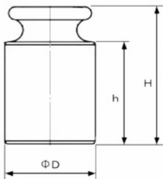
分銅外径図
