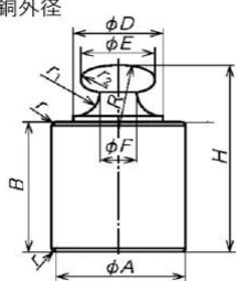
分銅外径図
