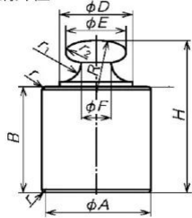
分銅外径図
