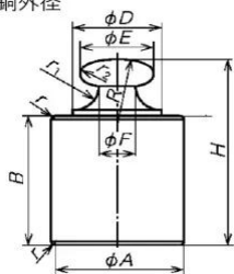
分銅外径図
