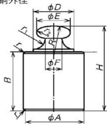
分銅外径図
