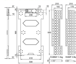
画像は、PADの寸法図です。
