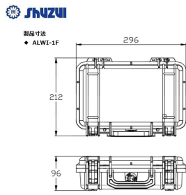
画像は、指示計：データBOXの寸法図です。
