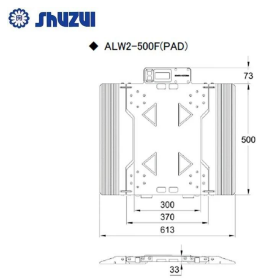
画像は、PADの寸法図です。
