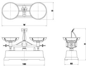
寸法図
