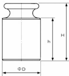
分銅外形図
