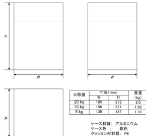
ケースサイズ寸法図
