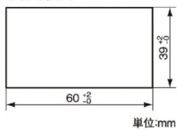
取付寸法図
