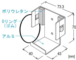
画像は、参考寸法図です。
