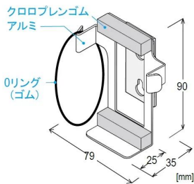
画像は、参考寸法図です。
