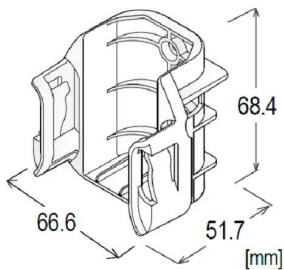
画像は、参考寸法図です。
